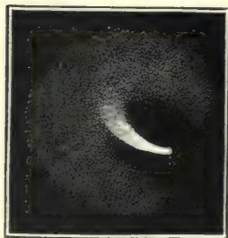
Aug. 22.
